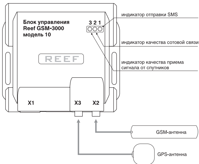
Рис. 8. Расположение индикаторов и разъемов блока управления системы
