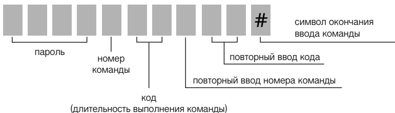
Рис. 2. Порядок отправки дополнительной команды
