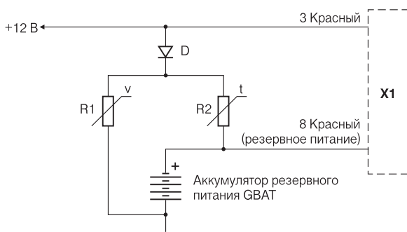
Рис. 11. Схема подключения источника резервного питания
