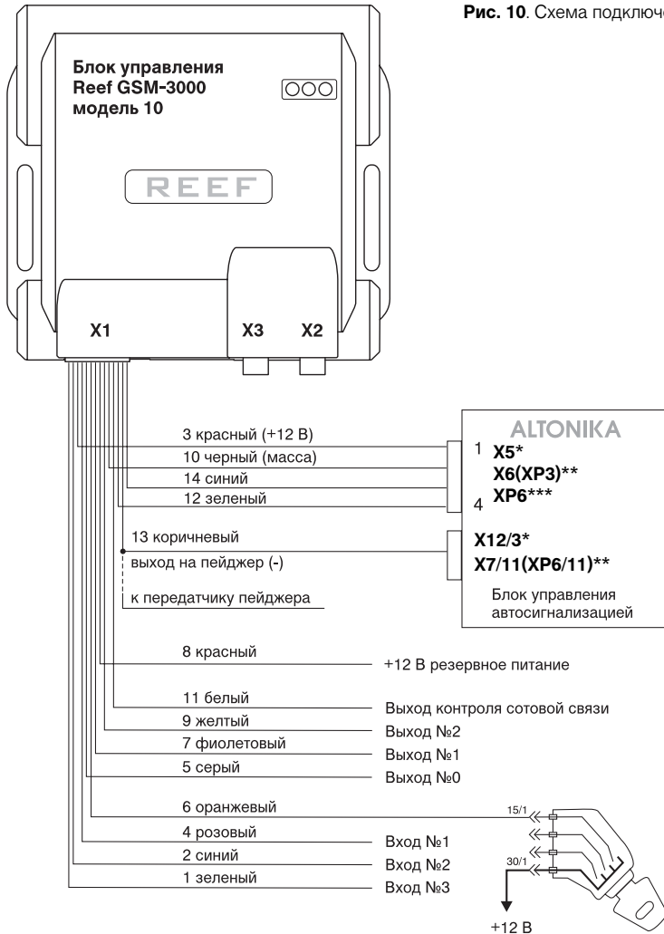
Рис. 10. Схема подключения
